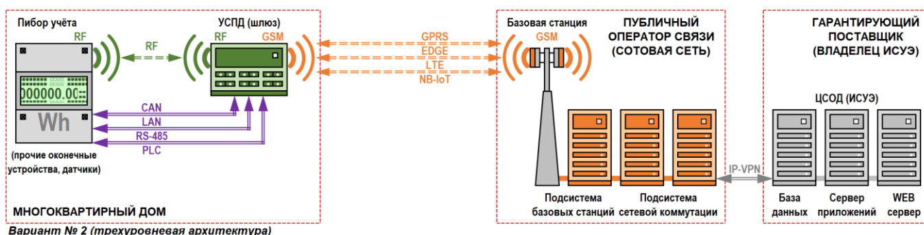
Рисунок № 1 Организация каналов (линий) связи на базе интерфейсов PLC и RF.
